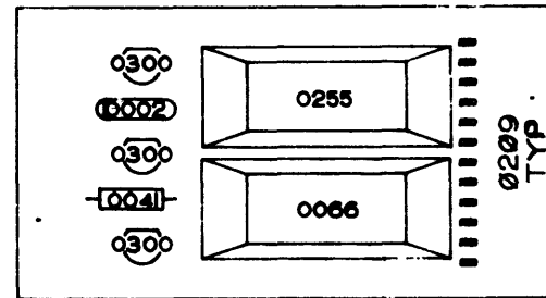
00300099001E2 LAYER 3
