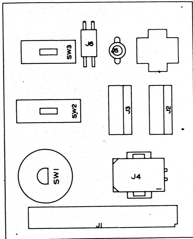
003000813-07 LAYER 5
