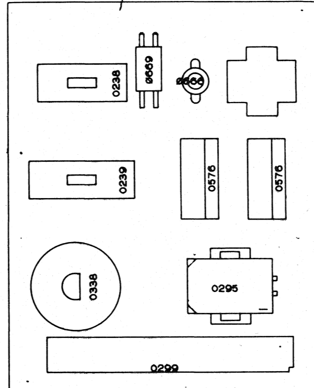
003000813-11 LAYER 3
